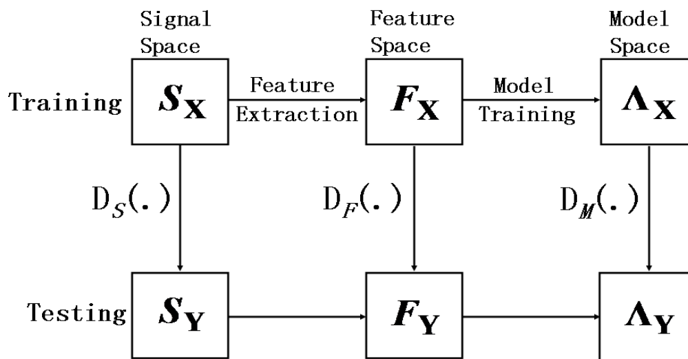
圖一：訓練與測試環境不匹配示意圖
