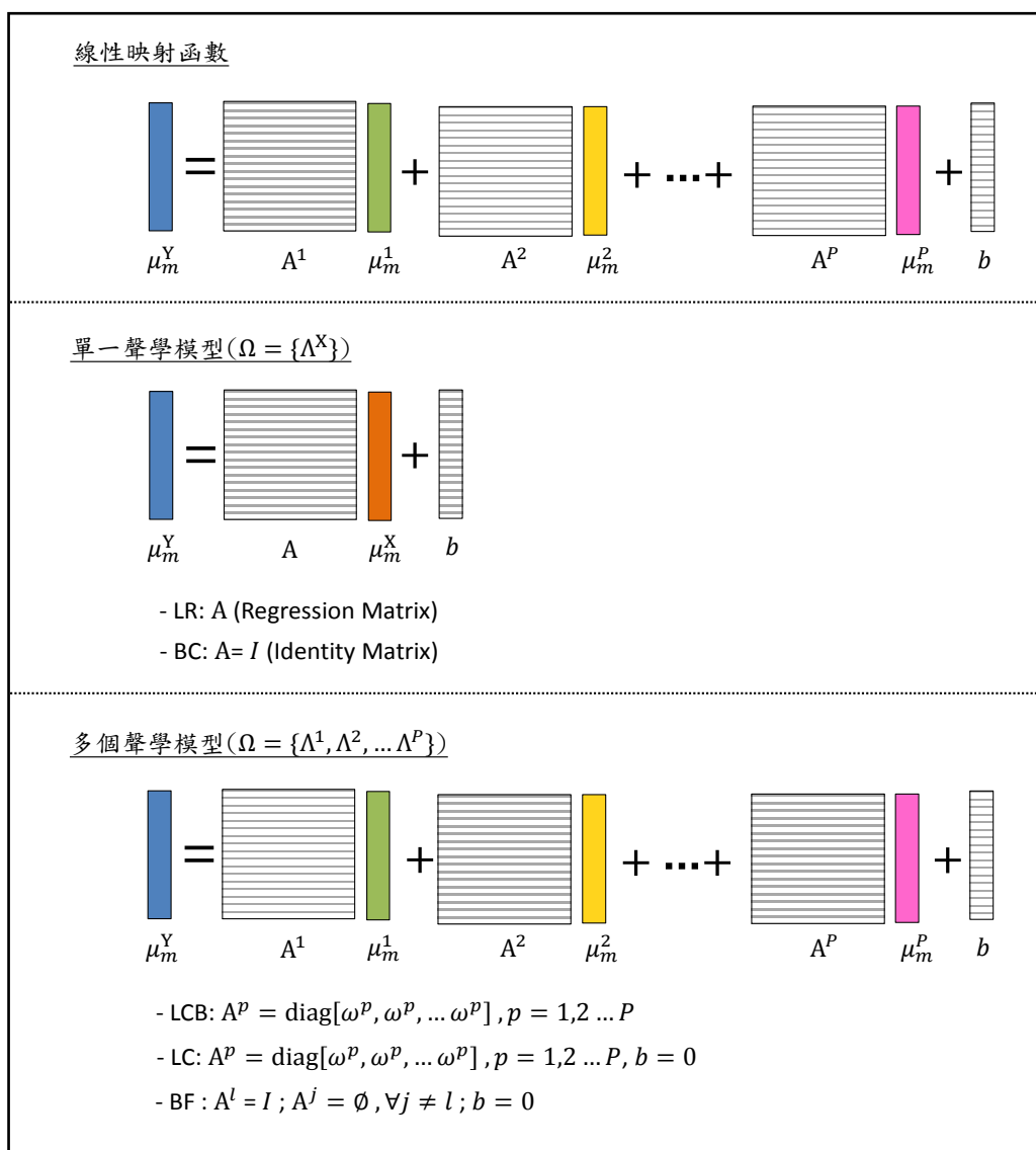
圖三：線性映射函數與其他轉換函數的比較
